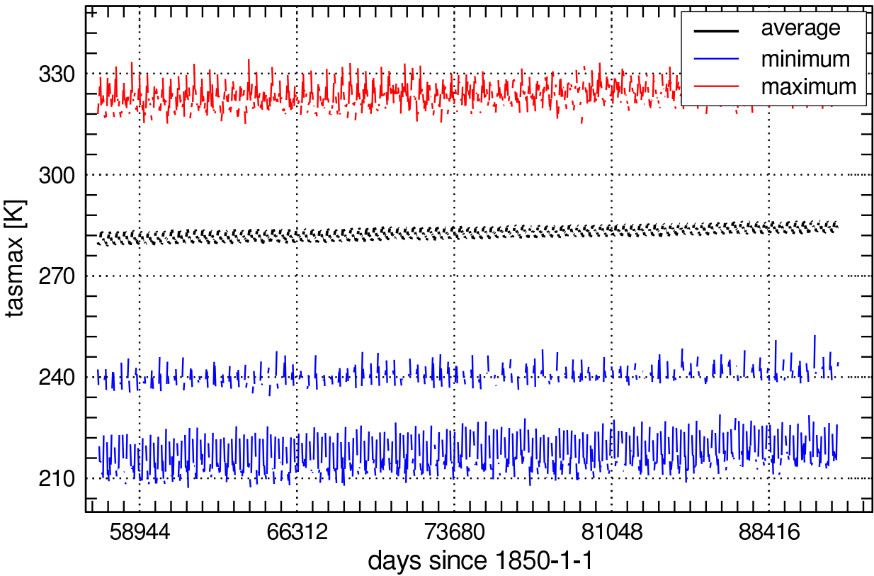
Global Values of tasmax_Amon
