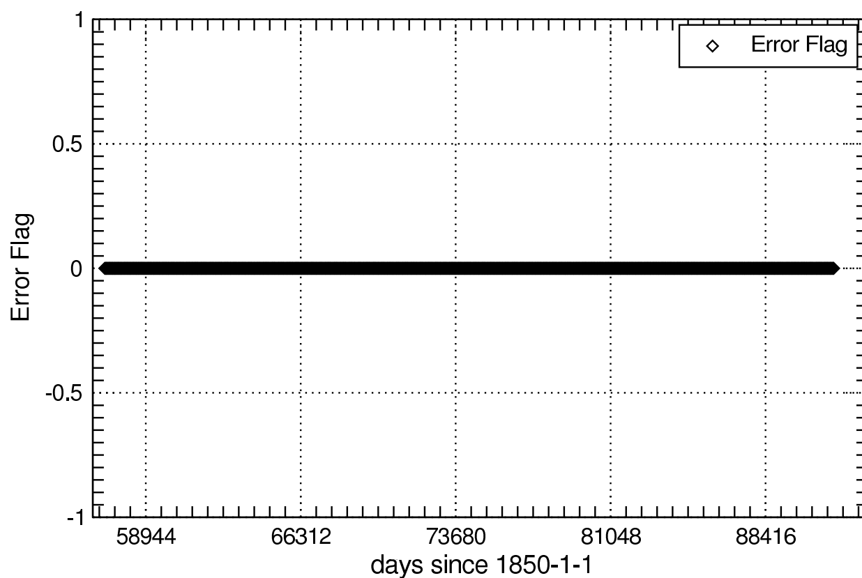
Error Flag of zossga_Omon
