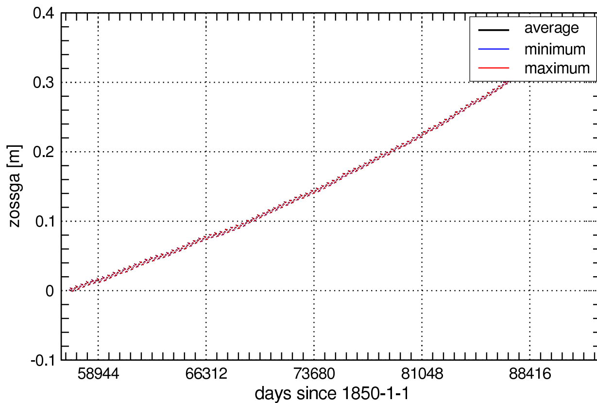
Global Values of zossga_Omon
