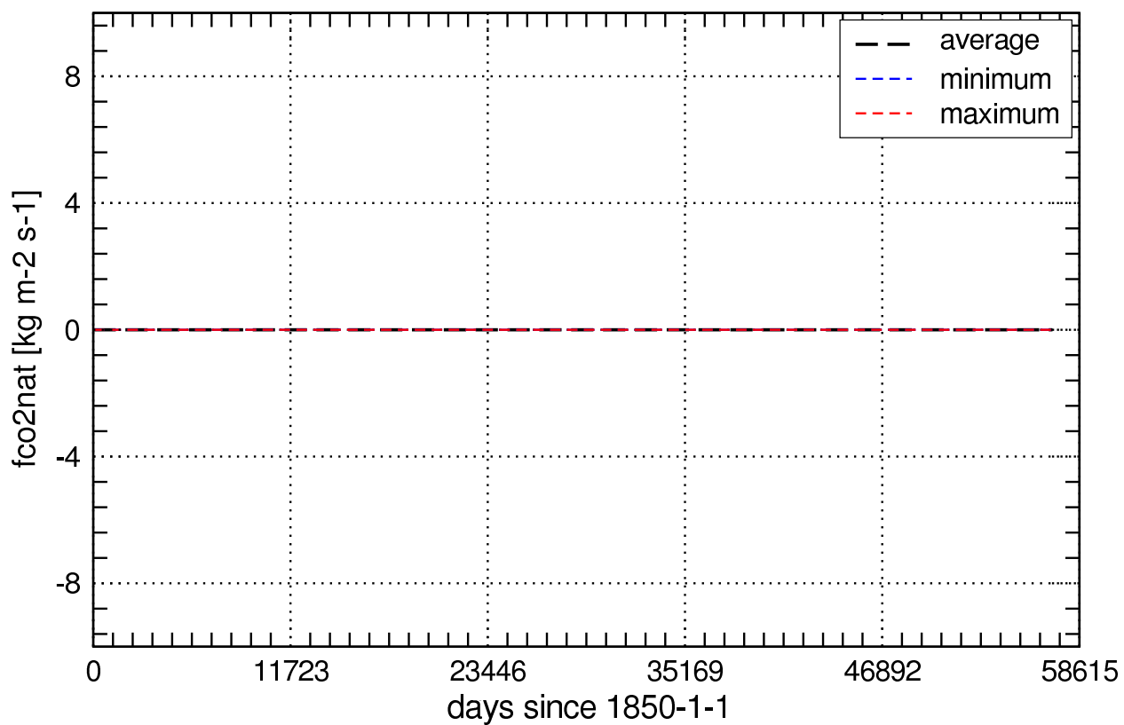
Global Values of fco2nat_Amon
