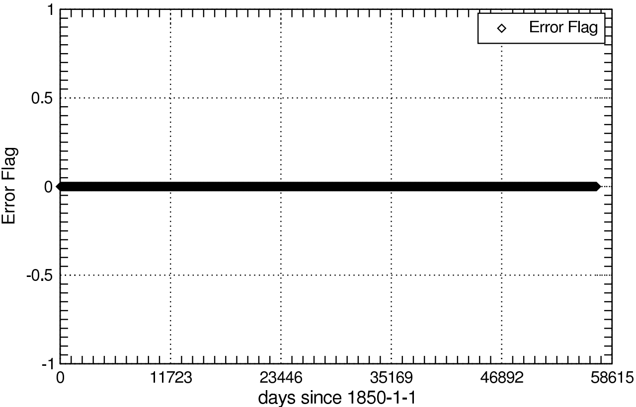
Error Flag of concso2_aero
