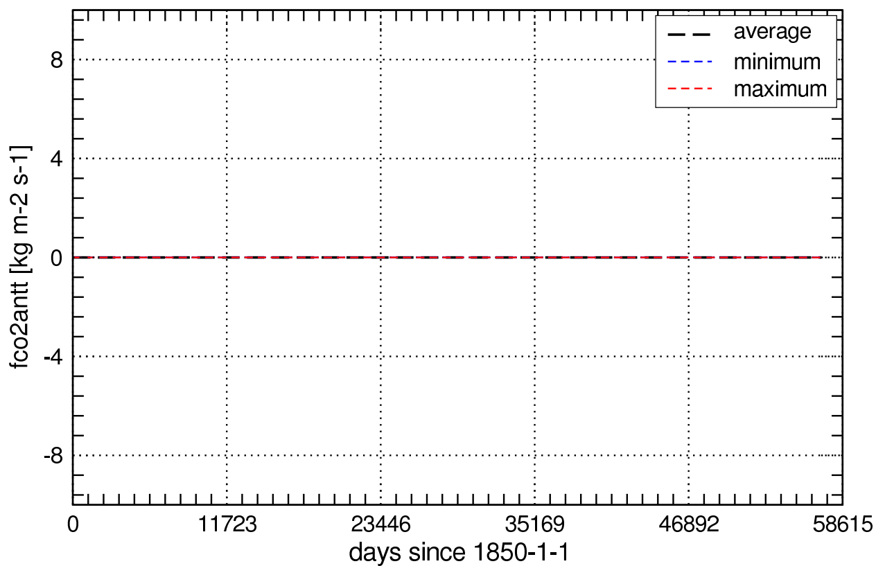
Global Values of fco2antt_Amon
