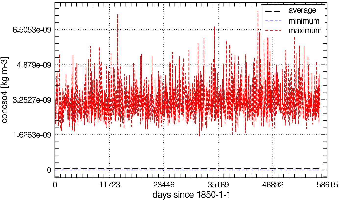
Global Values of concso4_aero
