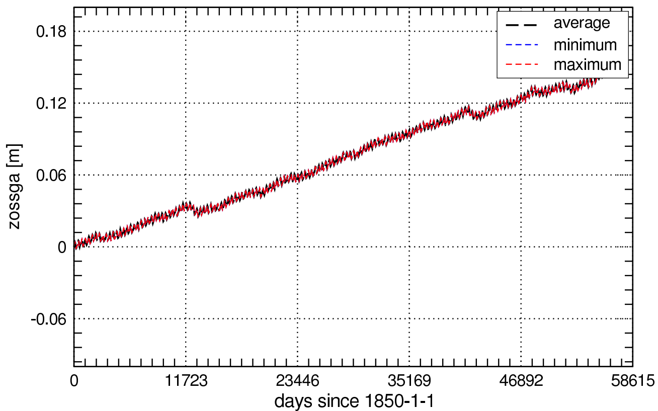
Global Values of zossga_Omon
