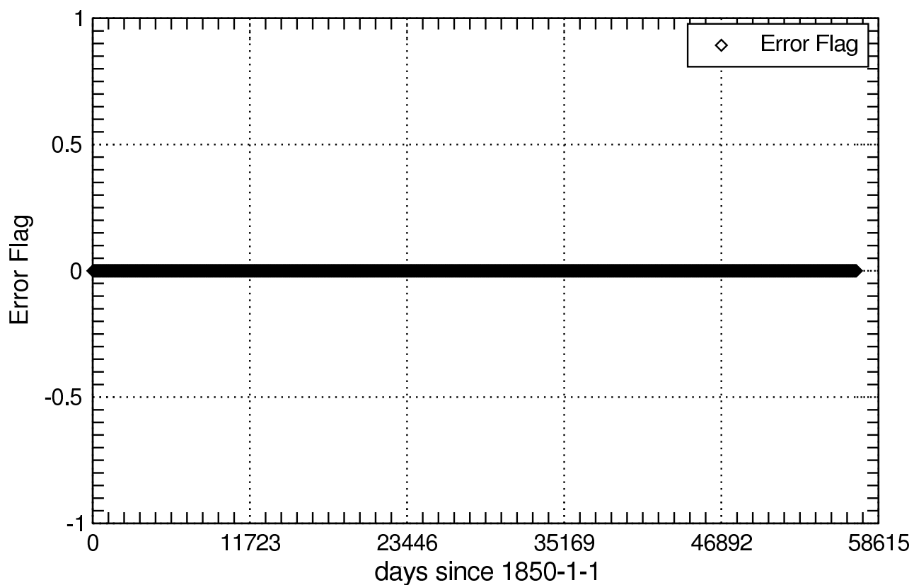
Error Flag of zossga_Omon
