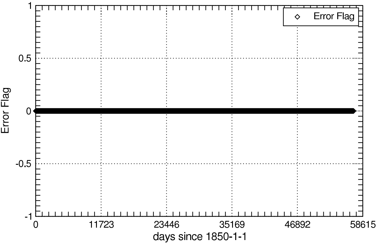
Error Flag of concso4_aero
