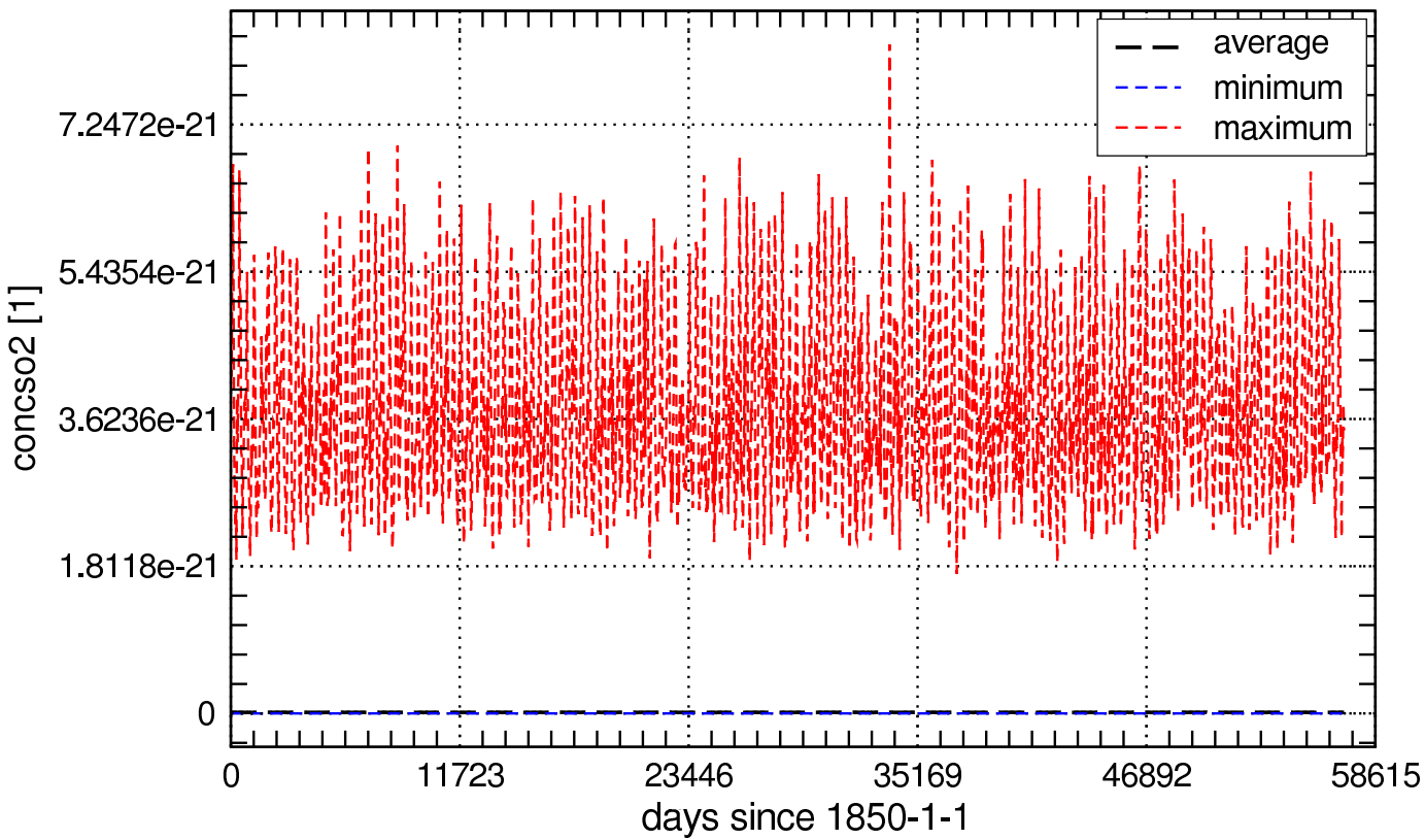
Global Values of concso2_aero
