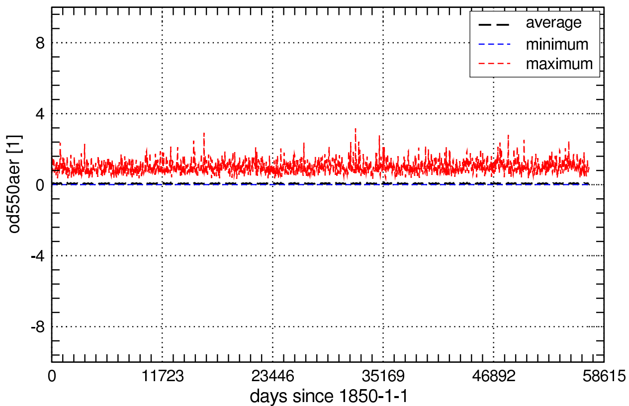
Global Values of od550aer_aero
