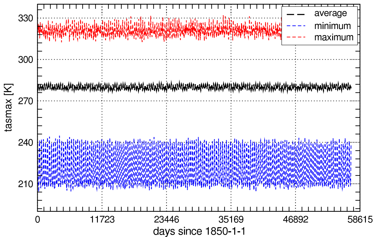
Global Values of tasmax_Amon
