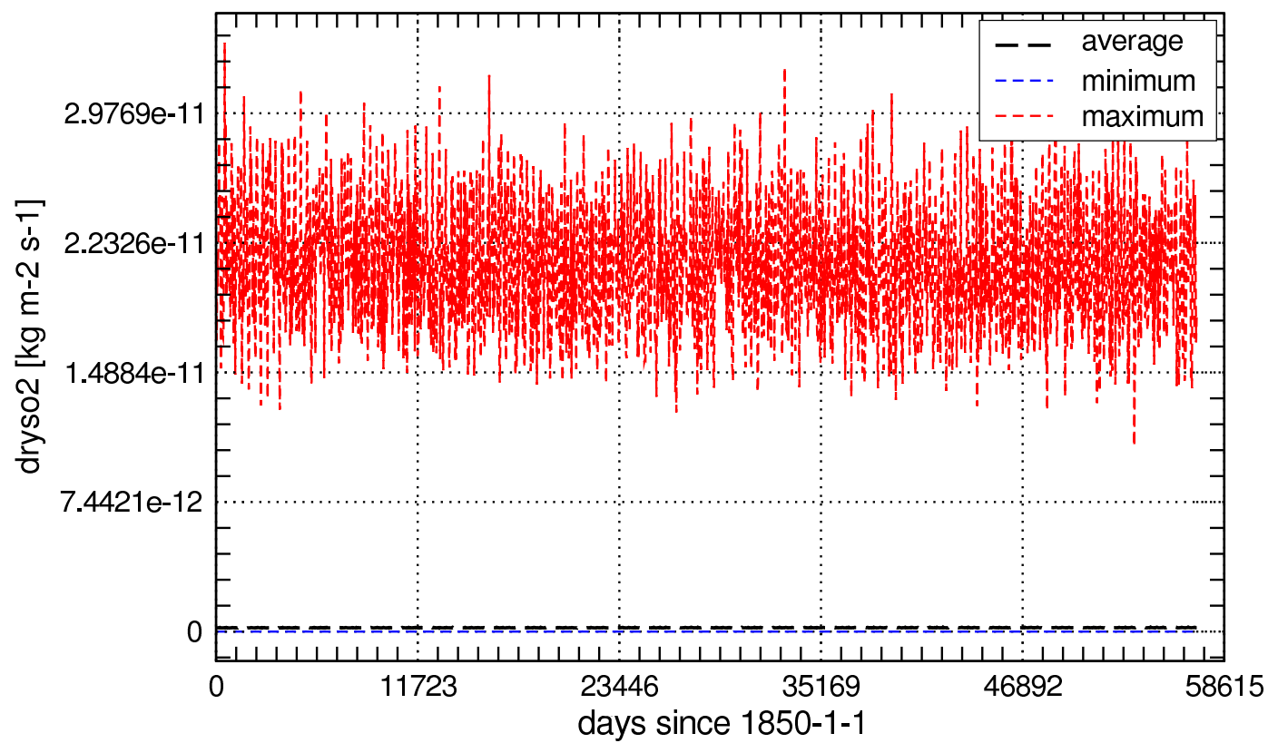
Global Values of dryso2_aero
