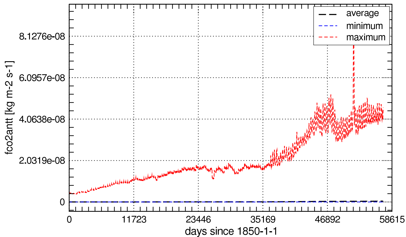
Global Values of fco2antt_Amon
