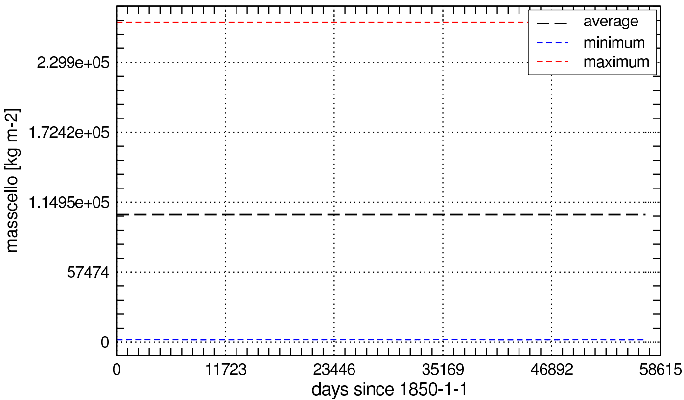
Global Values of masscello_Omon
