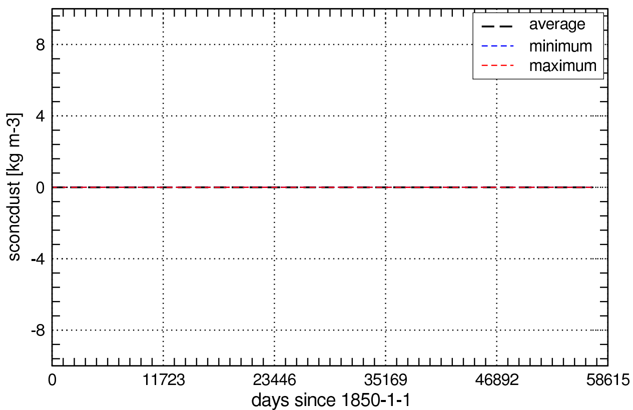
Global Values of sconcdust_aero
