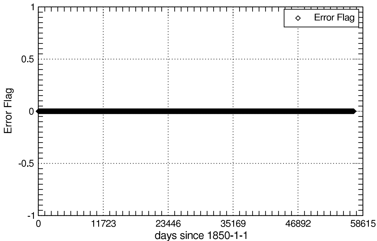
Error Flag of uas_Amon
