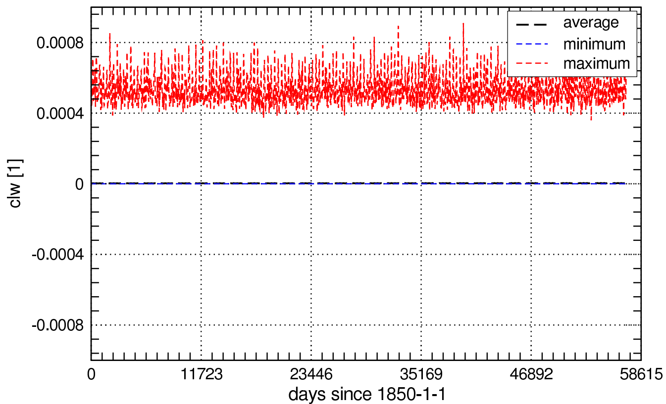
Global Values of clw_Amon
