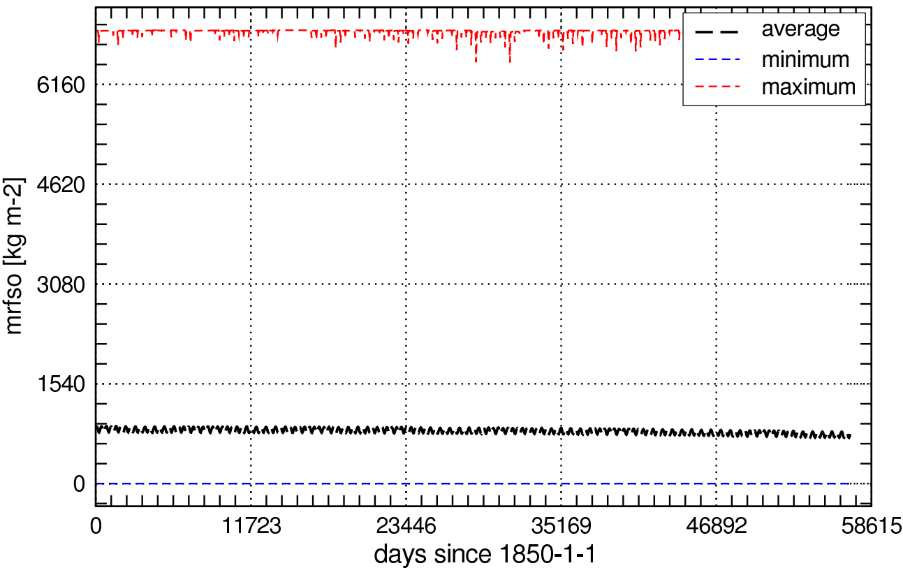
Global Values of mrfso_Lmon
