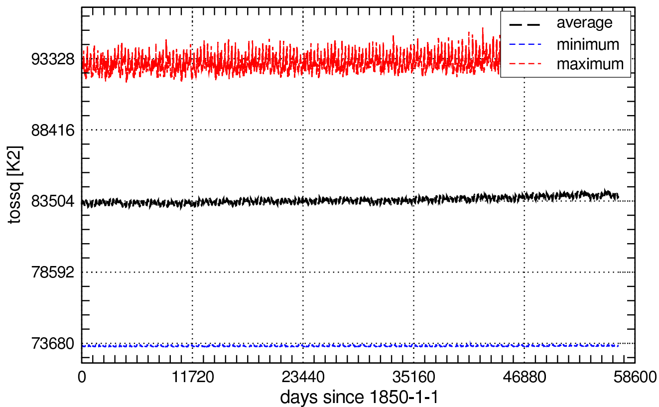
Global Values of tossq_day
