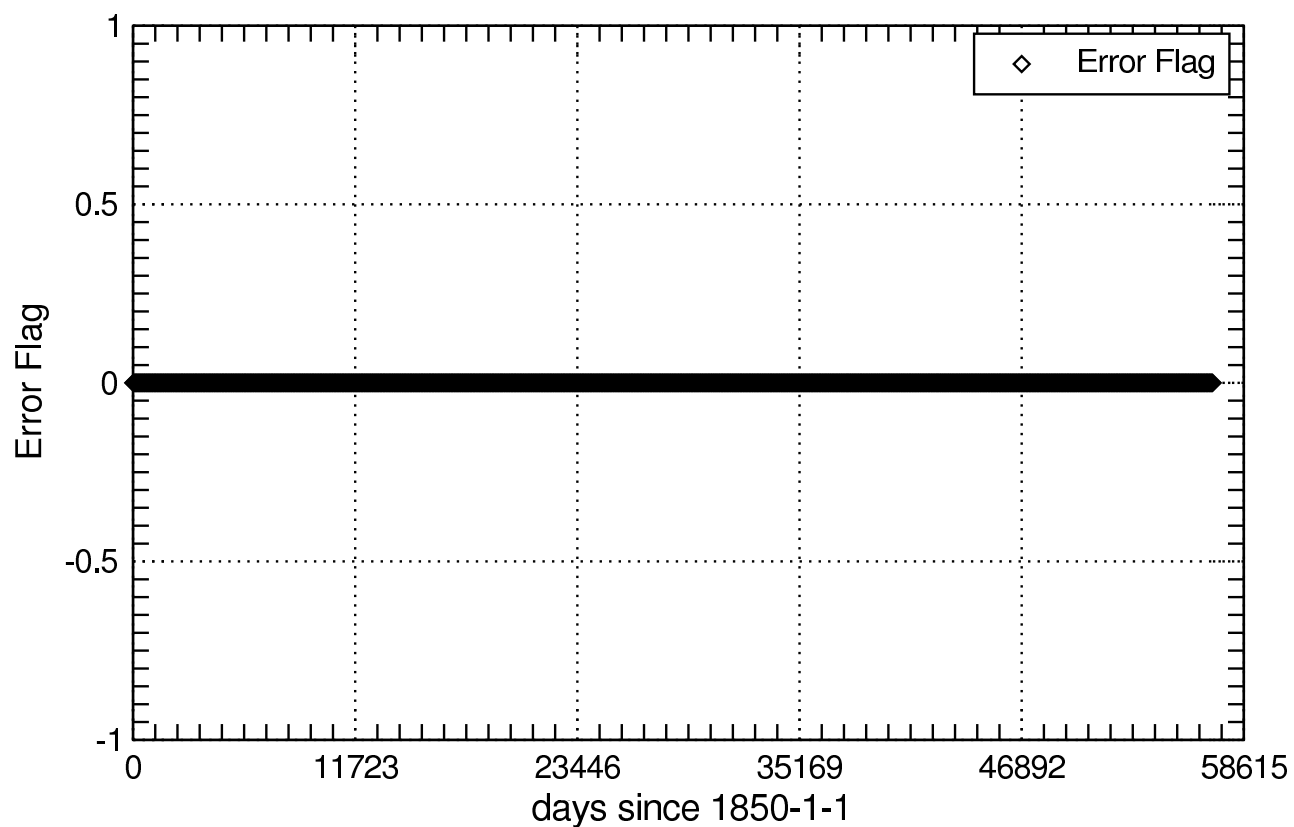
Error Flag of zostoga_Omon
