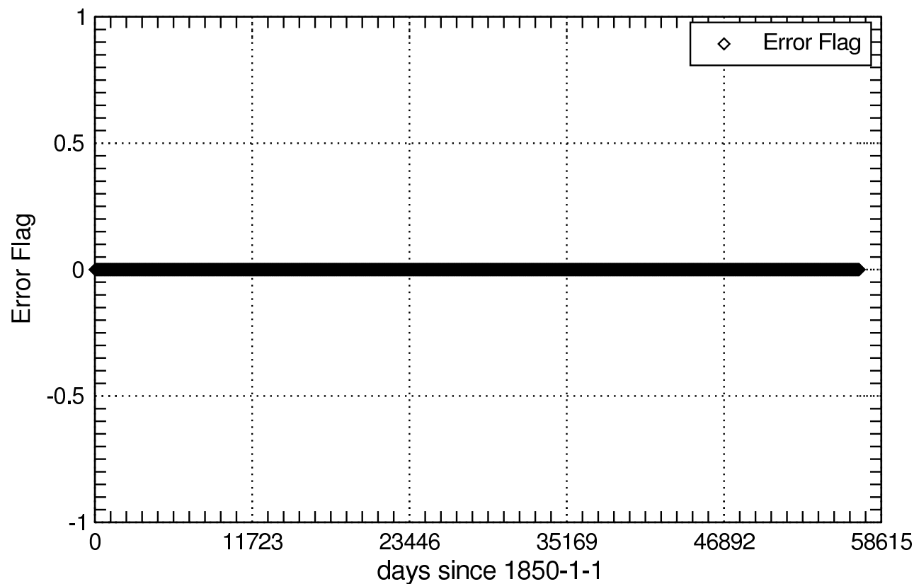
Error Flag of zos_Omon
