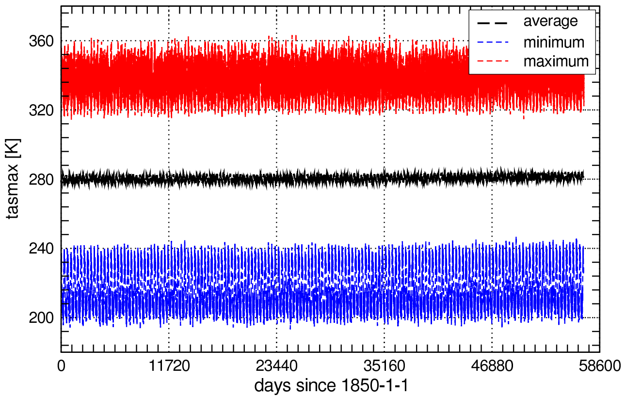
Global Values of tasmax_day
