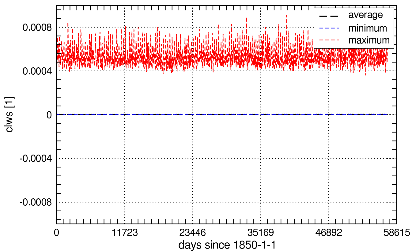
Global Values of clws_cfMon
