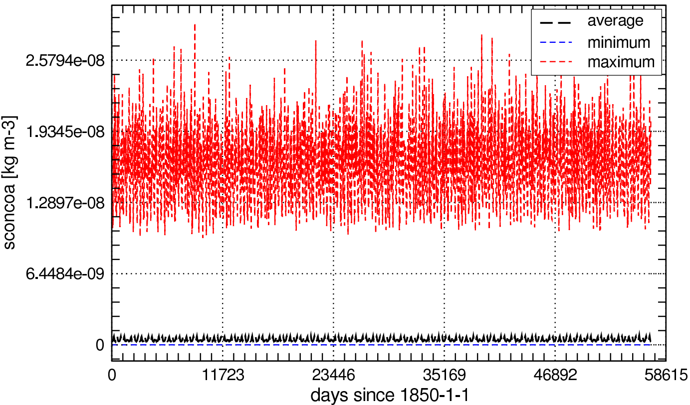
Global Values of sconcoa_aero
