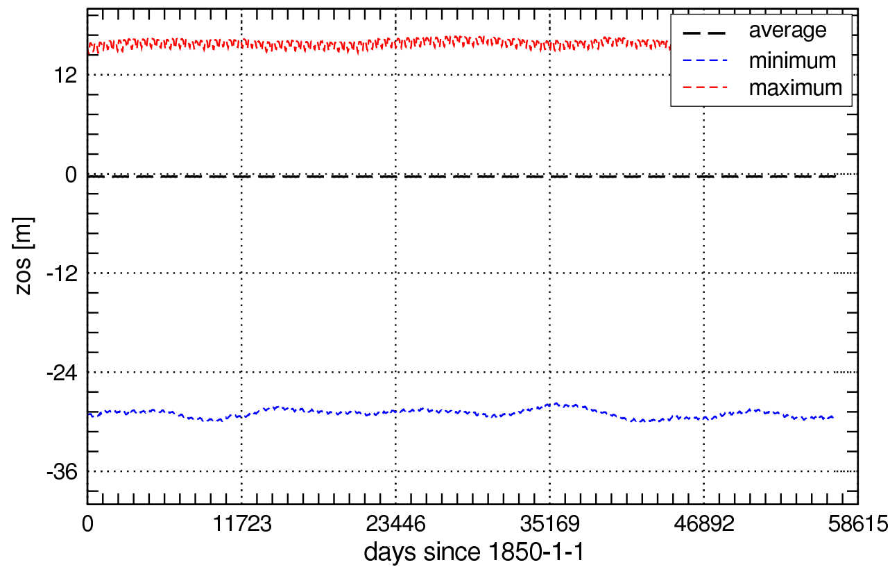
Global Values of zos_Omon
