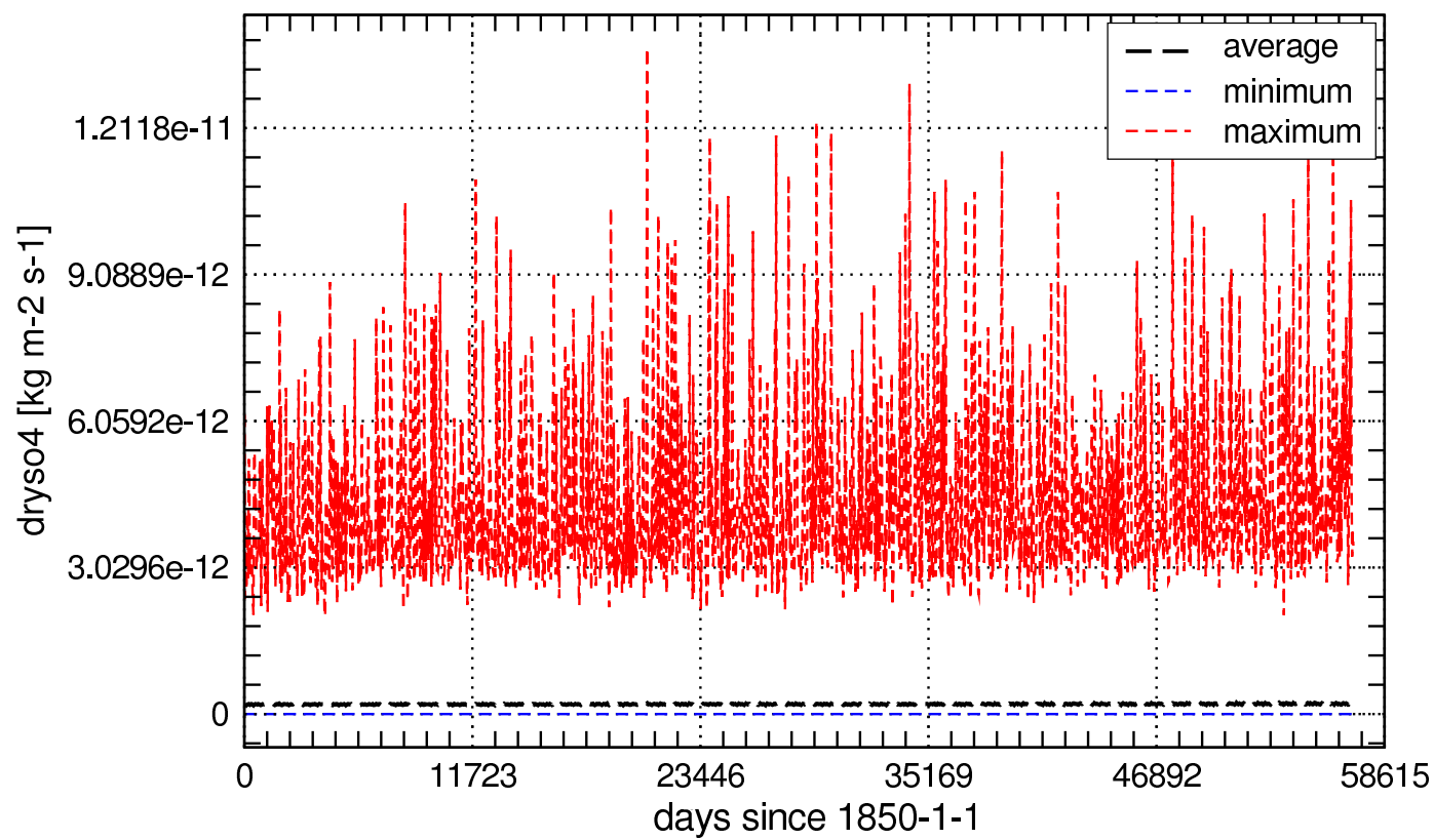
Global Values of dryso4_aero
