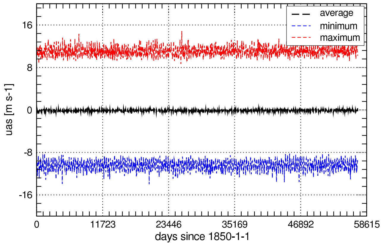
Global Values of uas_Amon
