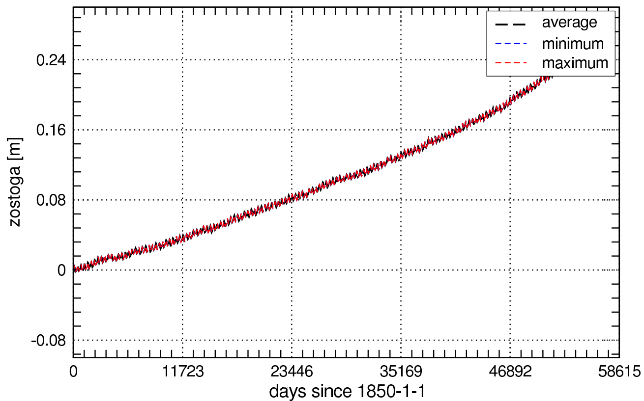
Global Values of zostoga_Omon
