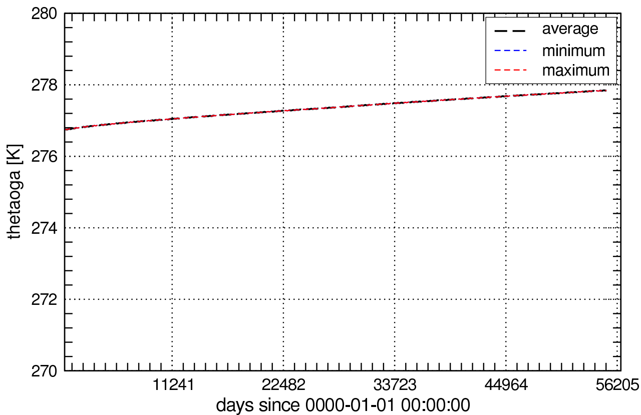
Global Values of thetaoga_Omon
