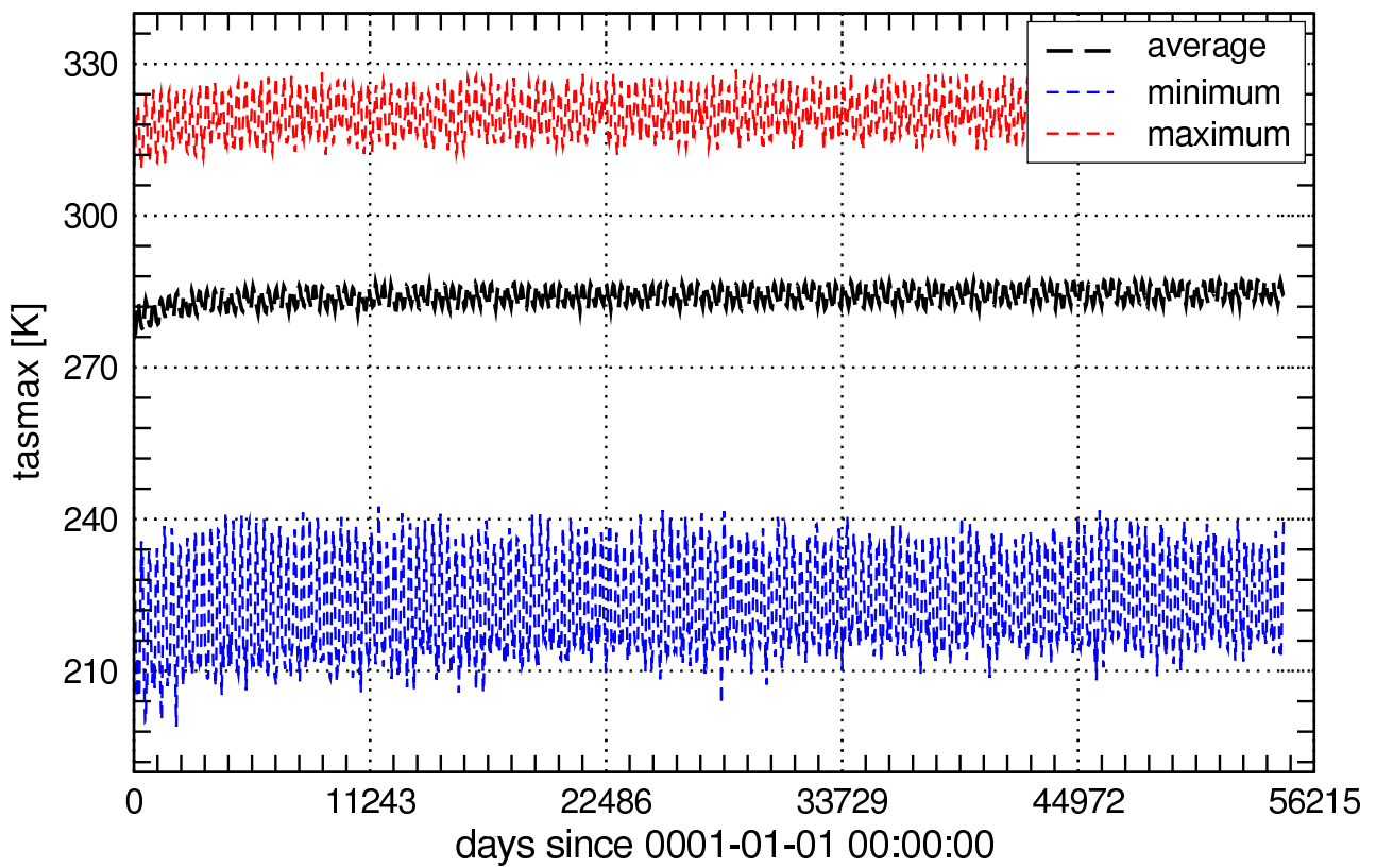
Global Values of tasmax_Amon
