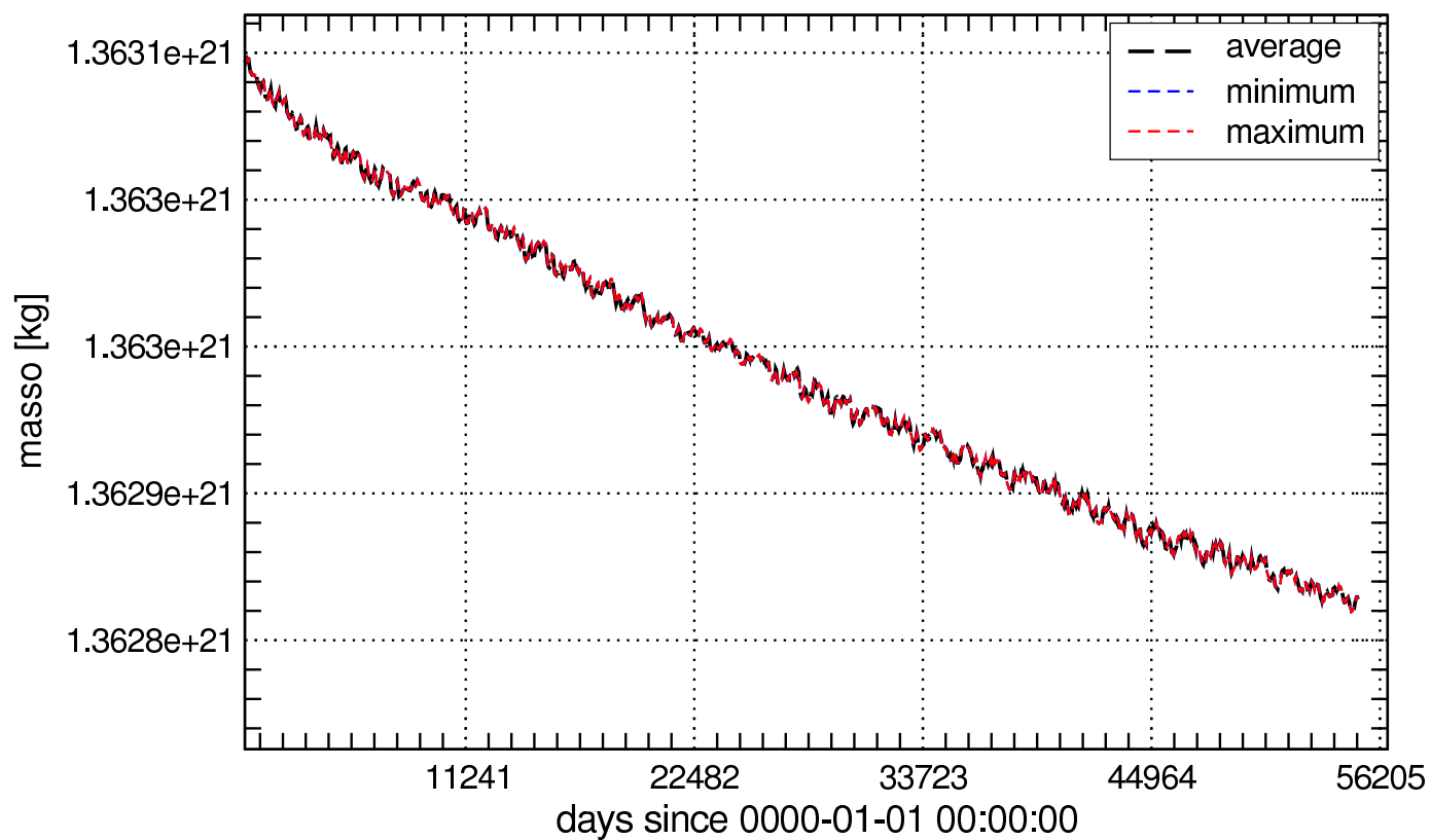
Global Values of masso_Omon
