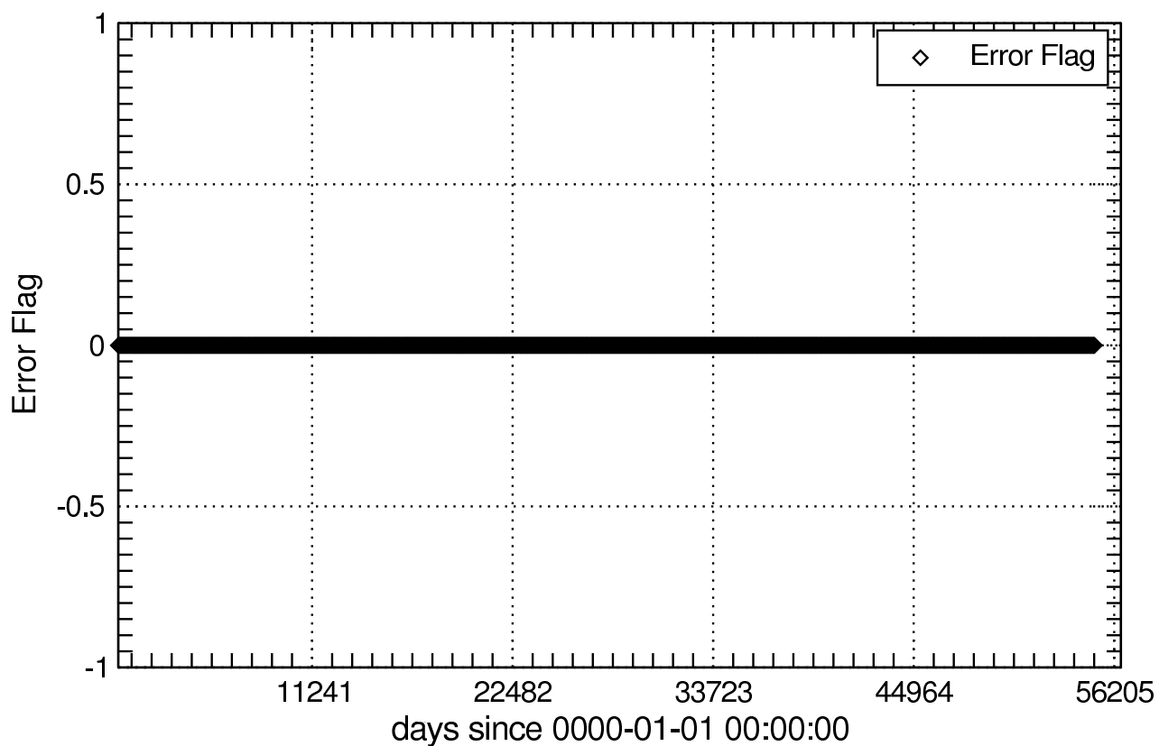
Error Flag of masso_Omon
