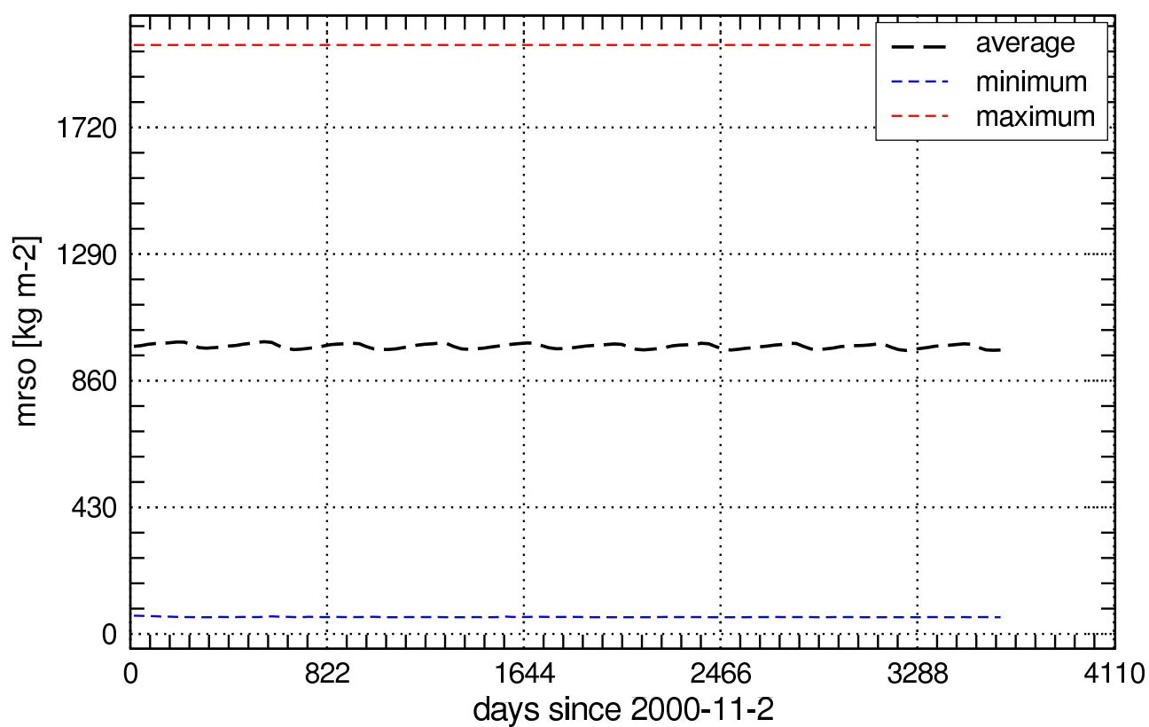
Error Flag of mrso_Lmon
