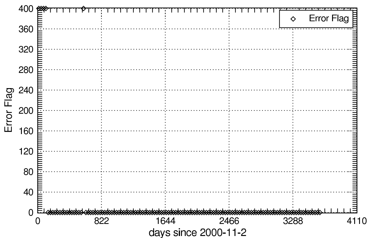
Error Flag of mrso_Lmon
