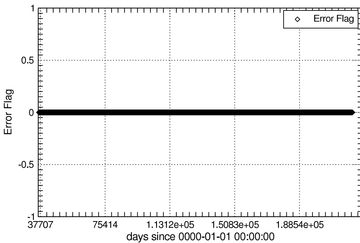
Error Flag of masso_Omon
